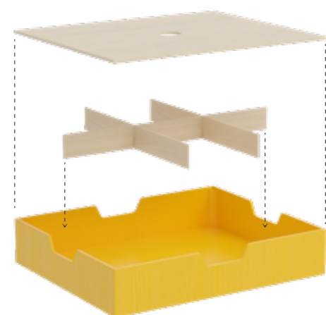
ДЕРЕВЯННЫЙ КОНТЕЙНЕР №1 С РАЗДЕЛИТЕЛЕМ И КРЫШКОЙ
