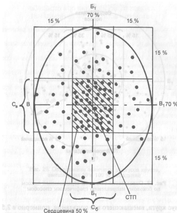
Рис. 27. Сердцевинные полосы и сердцевина рассеивания
