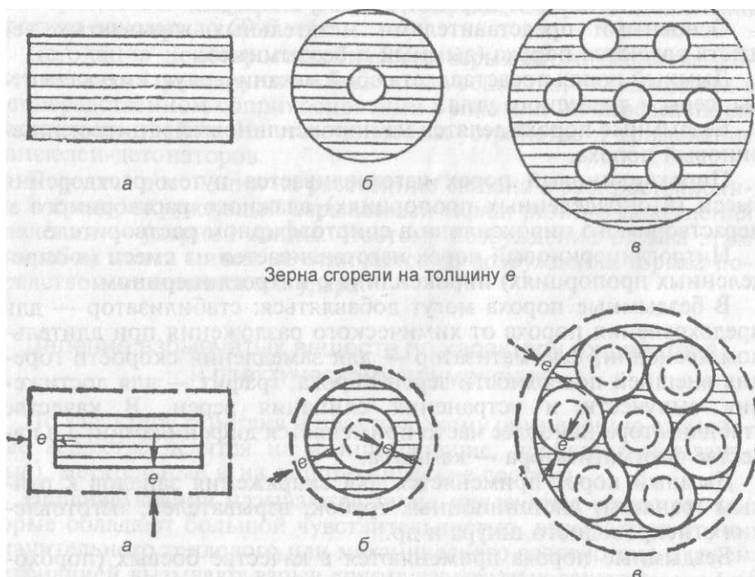
Рис. 49. Горение зерен бездымного пороха: а — депрессивной формы; б — с постоянной поверхностью горения; в — прогрессивной формы
