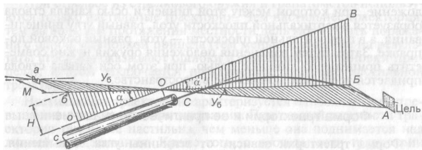
Рис. 13. Прицеливание (наводка) с помощью открытого прицела: O — мушка; a — целик; aO — прицельная линия; cC — ось канала ствола; oO — линия, параллельная оси канала ствола; Я — высота целика; М — величина перемещения целика; \alpha — угол прицеливания; \gamma_b — угол боковой поправки
