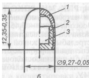
Рис. 131. 9-мм пистолетный патрон с пулей со стальным сердечником: а — патрон; б — пуля; 1 — оболочка; 2 — рубашка; 3 — сердечник стальной
