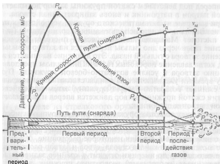
Рис. 1. Периоды выстрела:
