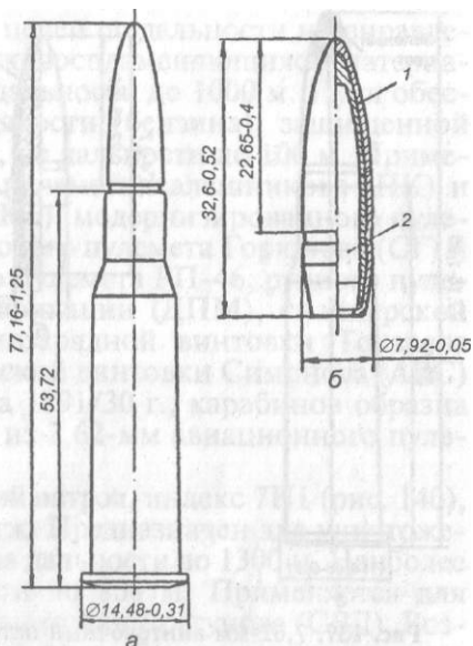
Рис. 136. 7,62-мм винтовочный патрон с пулей со стальным сердечником: а — патрон; 6 — пуля; 1 — оболочка; 2 — сердечник стальной
