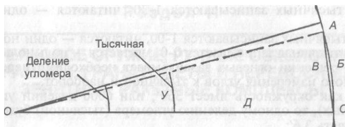
Рис. 50. Деление угломера и тысячная: ABC — дуга; AC — хорда
