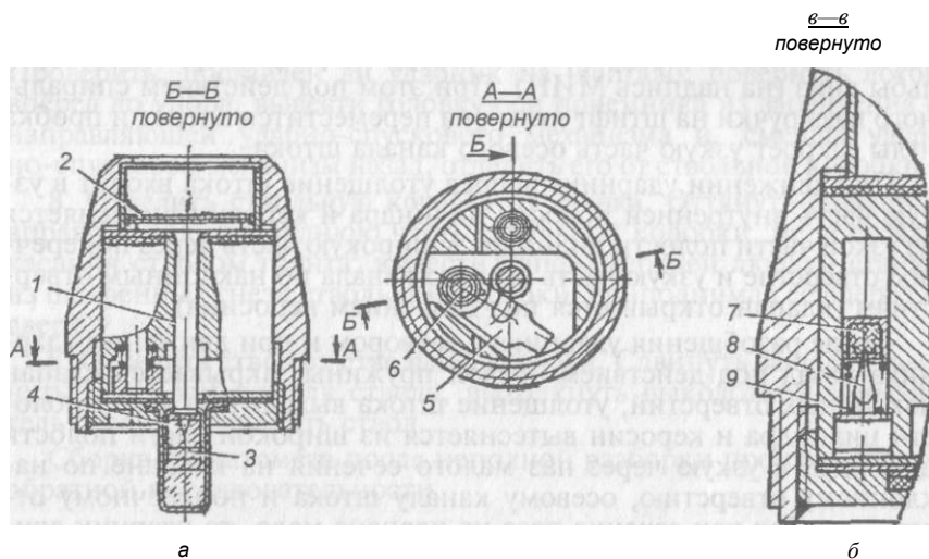
Рис. 106. Положение частей взрывателя:
