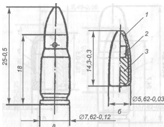
Рис. 127. 5,45-мм пистолетный патрон МПЦ: а — патрон; 6 — пуля; 1 — оболочка; 2 — сердечник стальной; 3 — сердечник свинцовый
