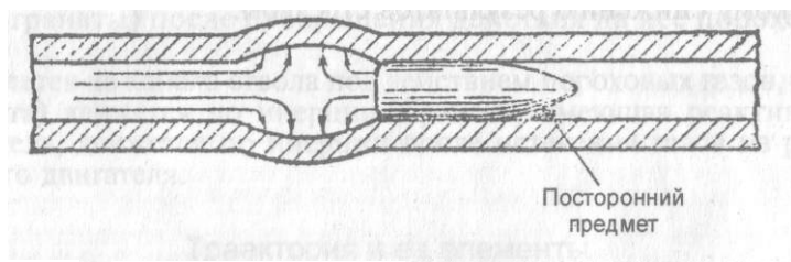
Рис. 4. Раздутие ствола
