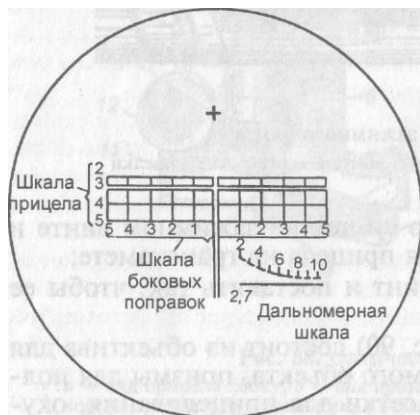
Рис. 91. Сетка оптического прицела РПГ-7
