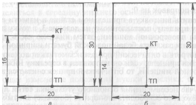
Рис. 148. Проверочные мишени:
