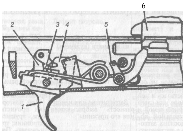
Рис. 73. Положение частей ударно-спускового механизма после одиночного выстрела: / — спусковой крючок; 2 — замедлитель курка; 3 — шептало одиночной стрельбы; 4 — курок; 5 — шептало автоспуска; 6 — затворная рама
